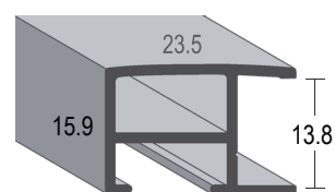
Profilserie 462-
