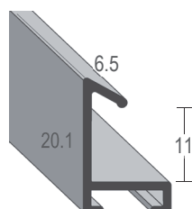
Profilserie 421-
