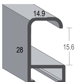
Profilserie 427-
