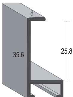
Profilserie 422-
