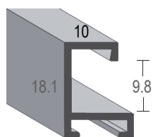
Profilserie 403-
