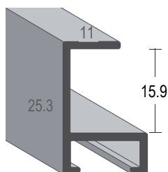
Profilserie 450-
