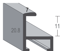
Profilserie 411-
