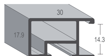
Profilserie 469-
