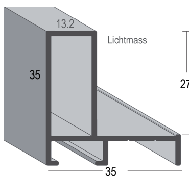
Profilserie 428-
