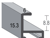
Profilserie 404-
