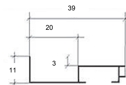
Profilschnitt
