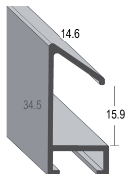
Profilserie 451-
