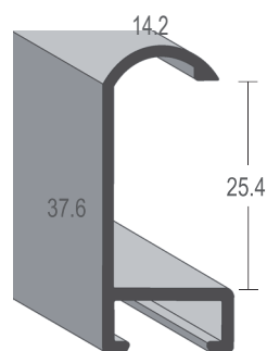
Profilserie 471-
